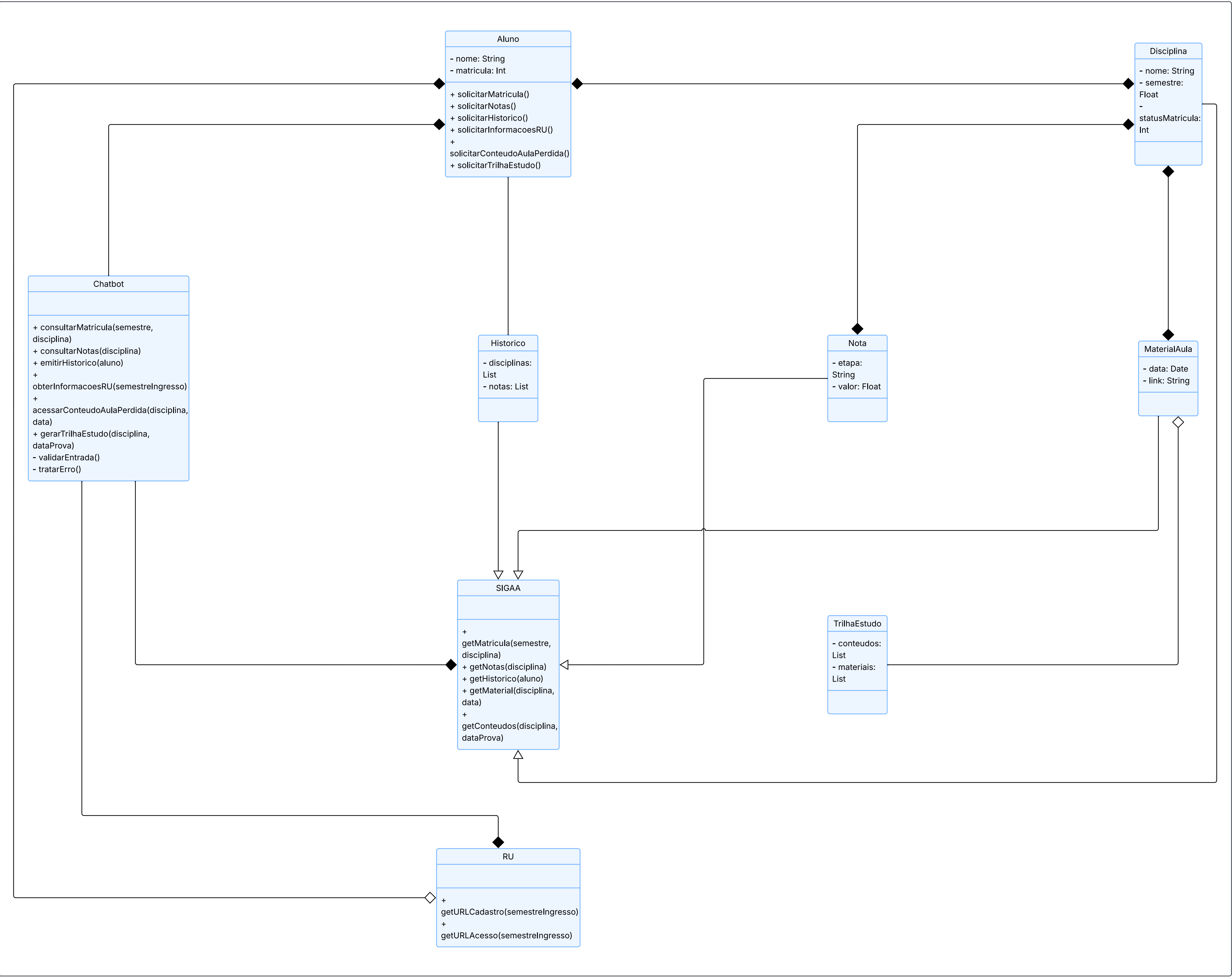
Diagrama de Classe do Sistema de Apoio Acadêmico
